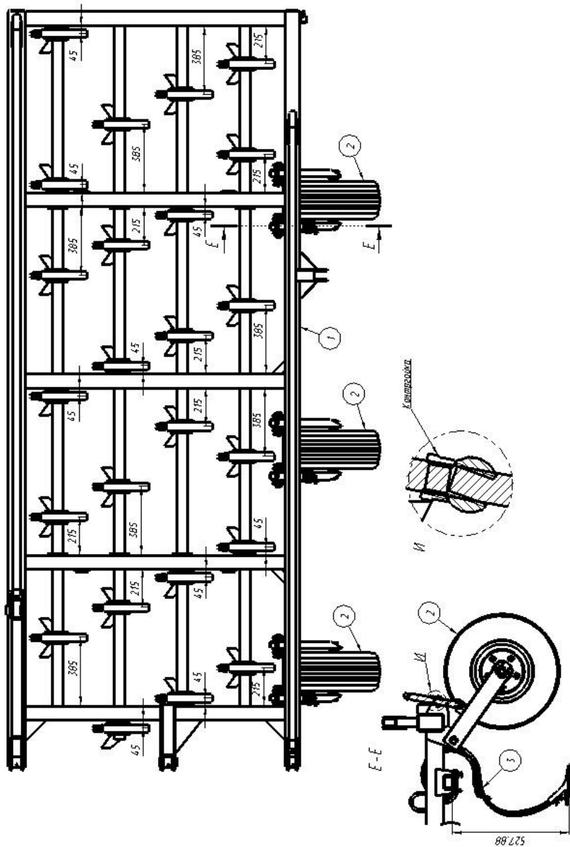
Рисунок 17 – Схема расстановки стоек 45x12 левого крыла КПМ-10Е
