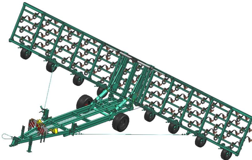
Рисунок 11 – Положение культиватора при развороте
