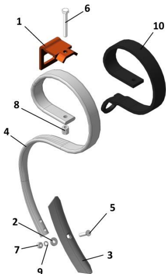
Рисунок 13 – КШЗ 00.050А Стойка с лапой
