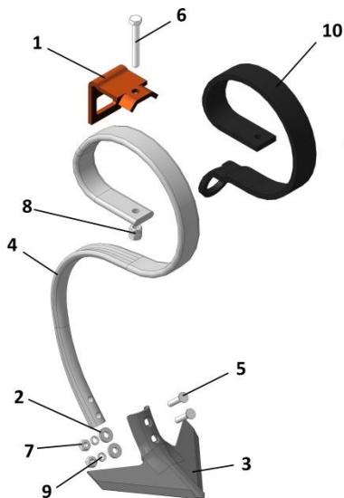
Рисунок 12 – КШЗ 00.050 Стойка с лапой
