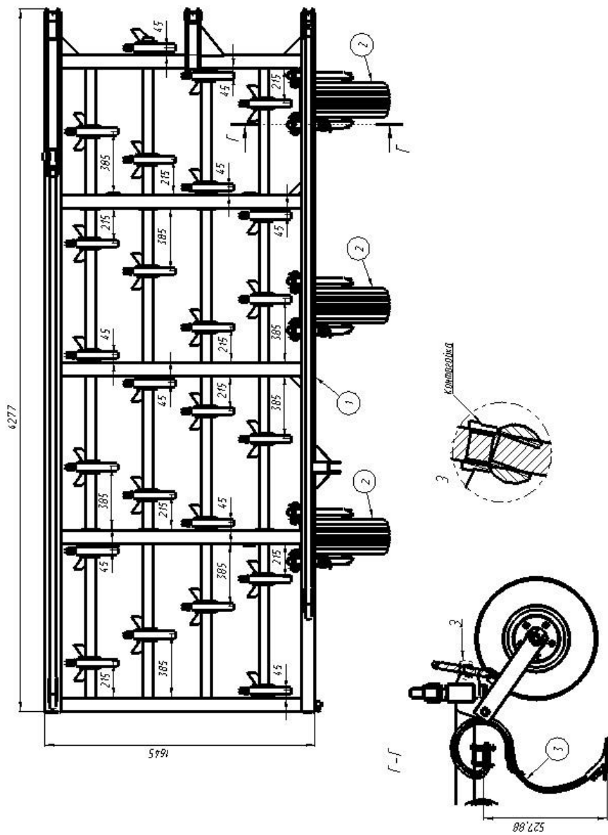
Рисунок 16 – Схема расстановки стоек 45x12 правого крыла КПМ-10Е
