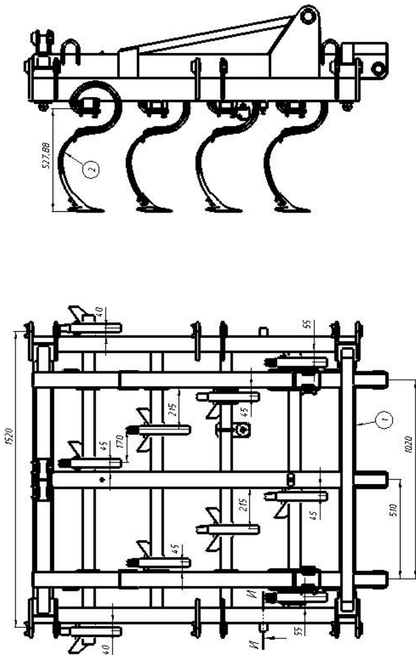
Рисунок 15 – Схема расстановки стоек 45x12 на центральной секции культиваторов КПМ-10Е и КПМ-12Е
