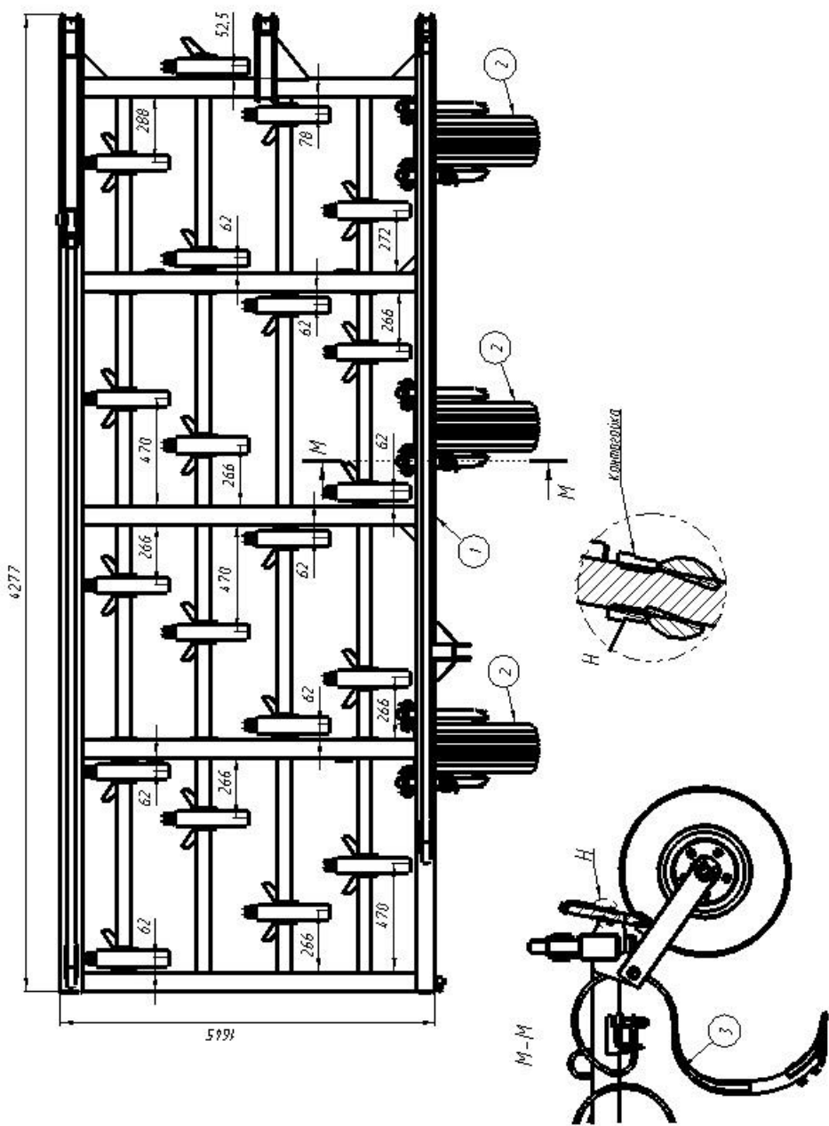
Рисунок 21 – Схема расстановки стоек 70x12 правого крыла КПМ-10Е
