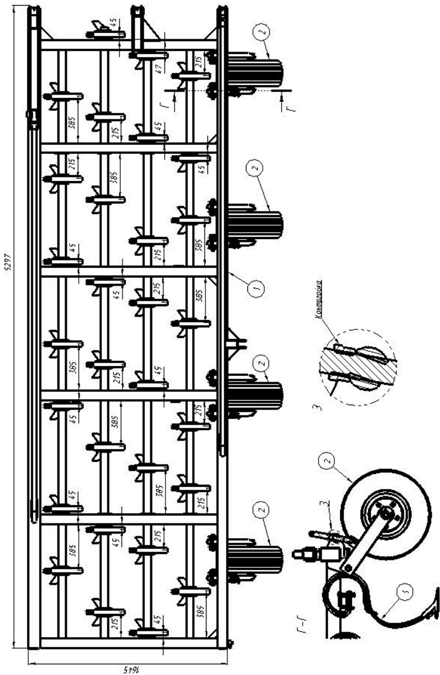
Рисунок 18 – Схема расстановки стоек 45x12 правого крыла КПМ-12Е
