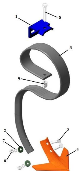
Рисунок 14 – КПМ 00.070 Стойка в сборе
