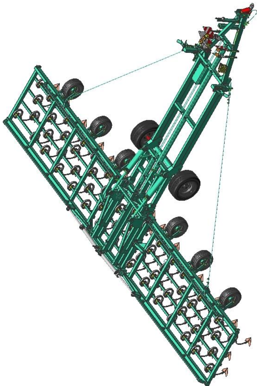
Рисунок 1а – Общий вид культиватора КПМ-10Е в рабочем положении (остальное см. рисунок 1)
